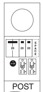
Fig. H R038CP4010 6-20R, (2) 5-20R2GFCI
