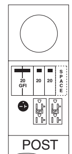
Fig. I R038CP4033 6-20R, (2) 5-20R2GFCI
