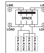
Fig. I U281E1P6H Series
