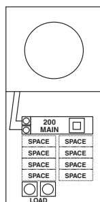
Fig. A M208CP6HP, R208CP6HP Series
