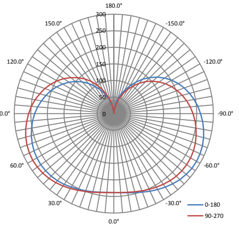
KT-LED20A21-O-E26-850-DIM
