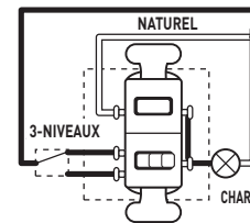
CABLE COMME VEILLEUSE
