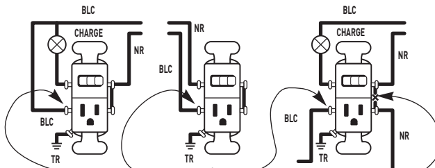
ALIMENTATION SEPARÉE (Plaquette de connexion retirée)
