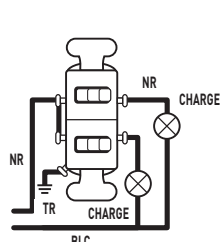
ALIMENTATION COMMUNE
