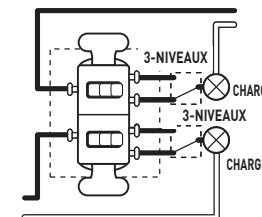
ALIMENTATION SEPARÉE (Langlette cassable retirée)
