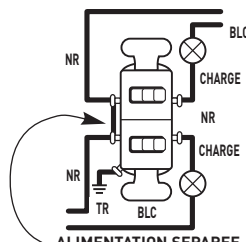
ALIMENTATION SEPARÉE (Plaquette de connexion retirée)
