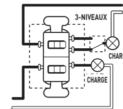
ALIMENTATION SEPARÉE (Langlette cassable retirée)
