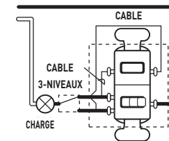
CABLE COMME LAMPE DE NUIT (Langlette cassable retirée)
