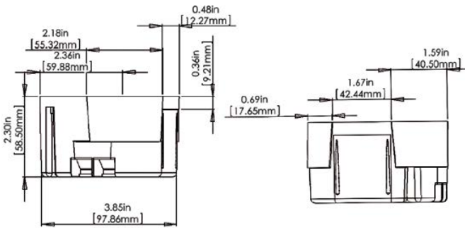
20 Cubic Inch Ceiling Fan Box
